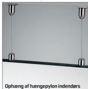
Ophæng af hængepylon indendørs
